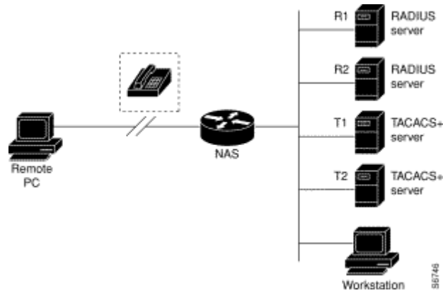
Figure Hata! Belgede belirtilen stilde metne rastlanmadı. -1 Typical AAA Network Configuration
